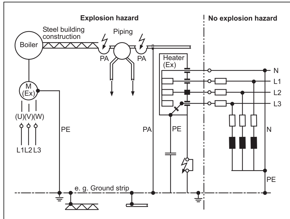
Fig. 14 Equipotential bonding in a hazardous area
