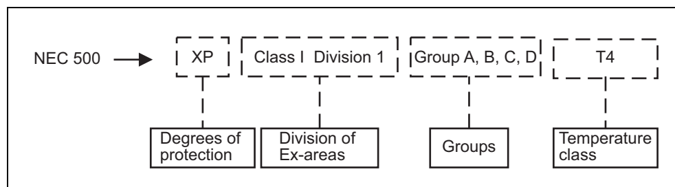
Fig. 5 NEC 500 overview
